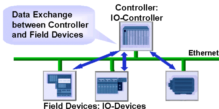
Rys 1: Architektura sieci PROFINet IO
