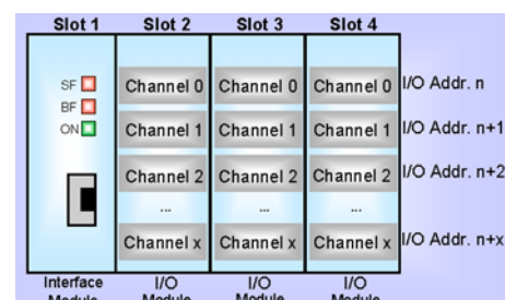
Rys 6: Model urządzenia dla PROFINet IO odpowiada modelowi PROFIBUS DP
