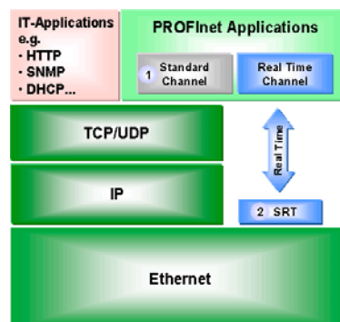
Rys 15: Kanały komunikacyjne PROFINet
