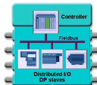
Rys 27: Metoda integracji aplikacji obiektowych
