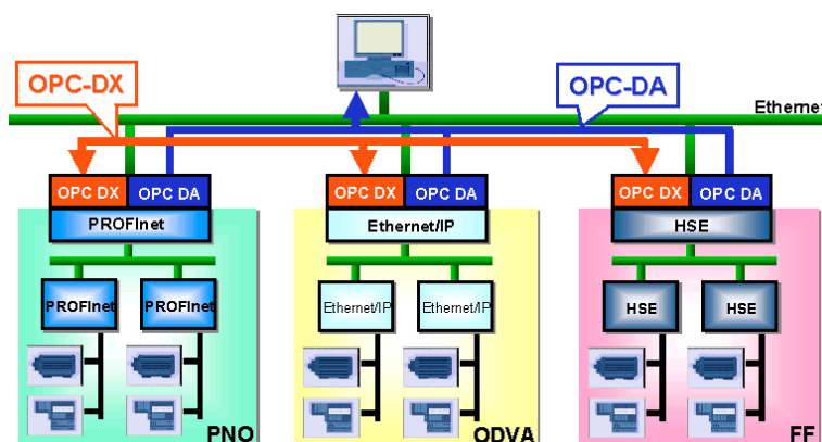
Rys 24: Wymiana danych pomiędzy systemami za pomocą OPC DA i OPC DX
