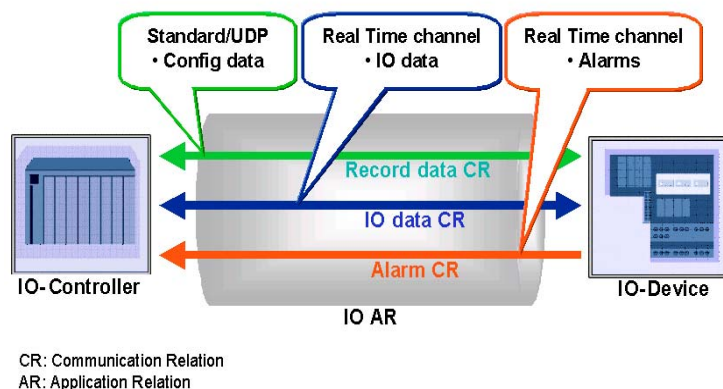
Rys 4: Powiązanie komunikacyjne dla PROFINet IO wg modelu Consumer/Provider
