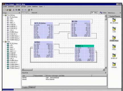
Rys 12: Widok obiektów w edytorze połączeń
